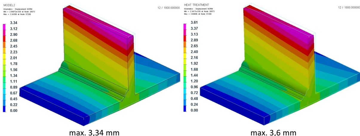
Rys. 5. Rozkład odkształceń całkowitych po procesie obróbki cieplnej złącza spawanego bez podgrzewania wstępnego (po lewej) oraz z podgrzewaniem wstępnym do 150°C (po prawej), tabl. V
