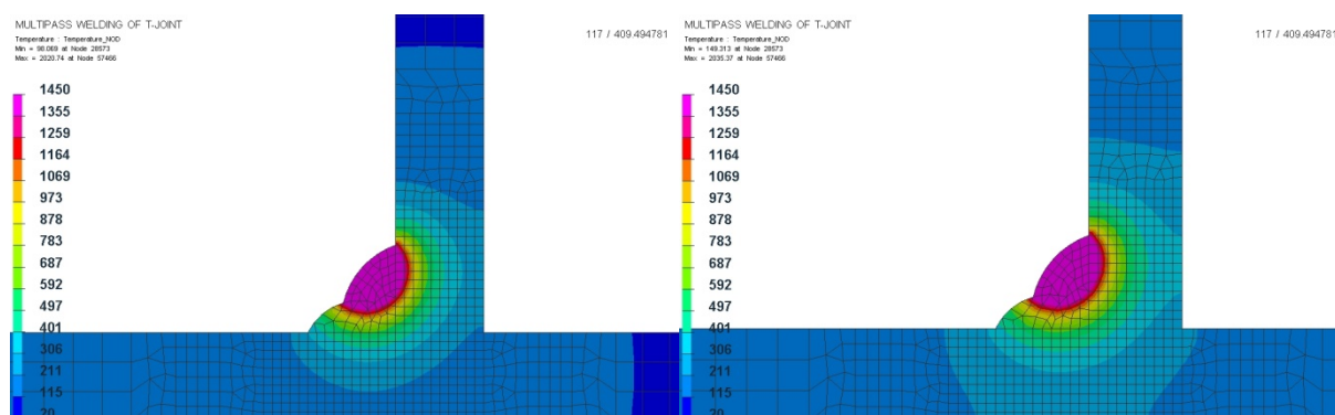
Rys. 2. Przykładowy rozkład temperatur w trakcie spawania 3-go ściegu na przekroju poprzecznym złączy teowych blach o grubości 10 mm ze stali S355J2G3 metodą MAG bez podgrzewania wstępnego (po lewej) oraz z podgrzewaniem wstępnym do 150°C (po prawej)
