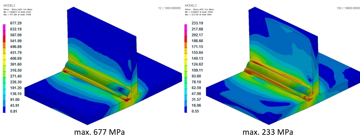
Rys. 6. Rozkład naprężeń zredukowanych (VonMises) po procesie spawania oraz obróbki cieplnej złączy teowych blach o grubości 10 mm ze stali S355J2G3 metodą MAG spawanego bez podgrzewania wstępnego, tabl. VI
