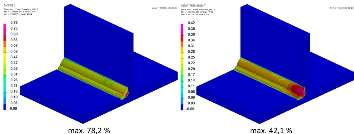
Rys. 4. Rozkład martenzytu odpuszczonego po procesie obróbki cieplnej (odpuszczania w temperaturze 600°C) złączy teowych blach o grubości 10 mm ze stali S355J2G3 metodą MAG spawanych bez podgrzewania wstępnego (po lewej) oraz z podgrzewaniem wstępnym do 150°C (po prawej), tabl. III
